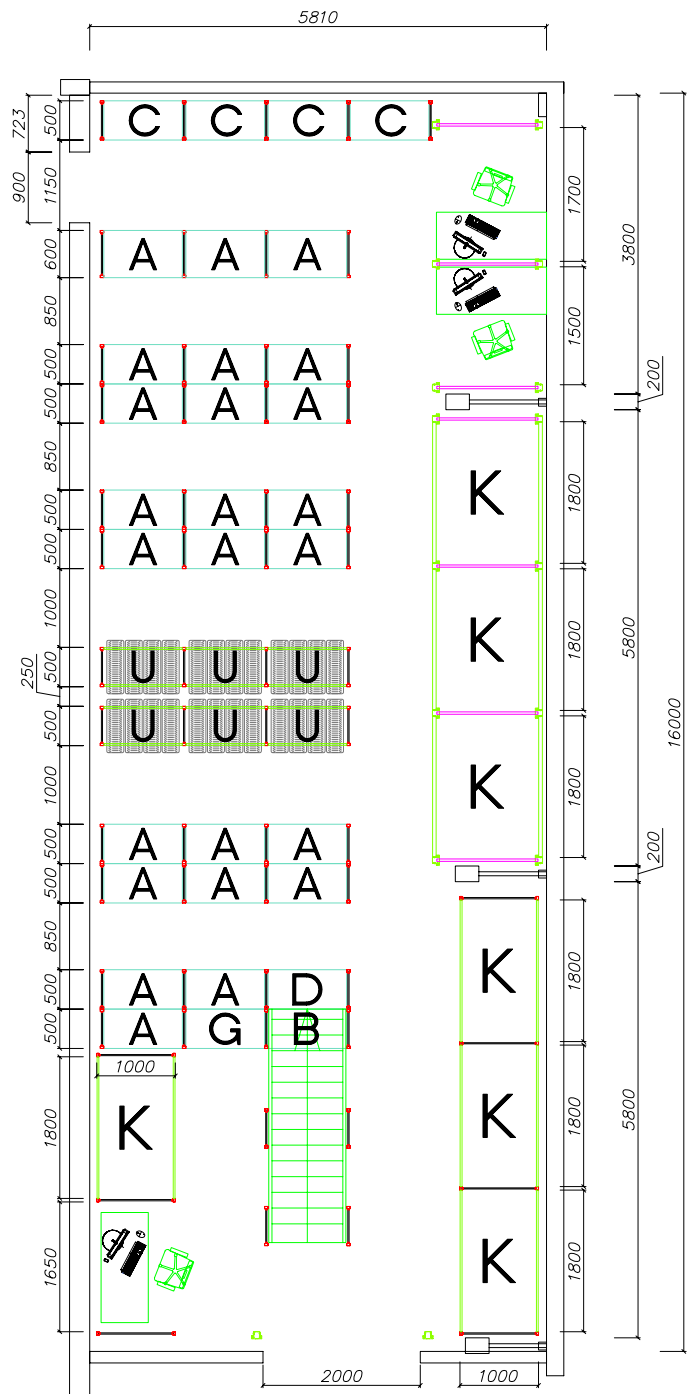
План на отм. +0.000
