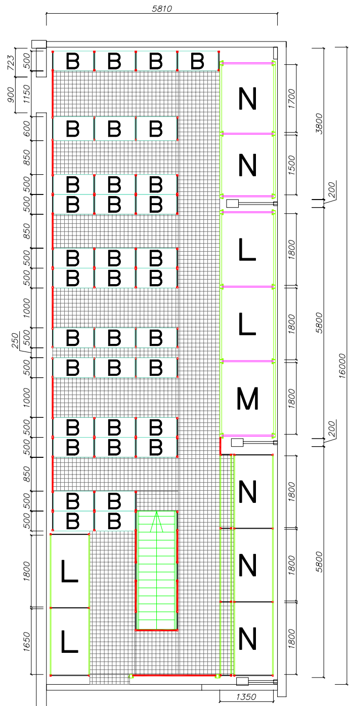
План на отм. +2.550
